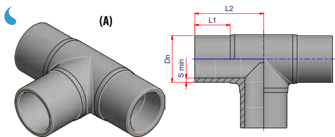
ТРОЙНИК 90° С УДЛИНЕННЫМИ ПАТРУБКАМИ (SDR 11)
